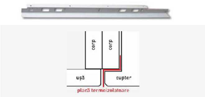
fig. 1 - PLACĂ PENTRU DIRIJAREA CĂLDURII
